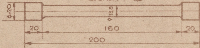
TRACÇÃO - CORPOS DE PROVA B-4e B-5 ESCALA 1:25
