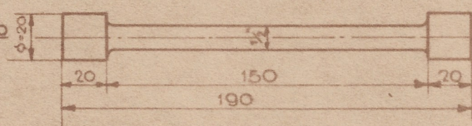
TRACÇÃO - CORPOS DE PROVA B-4e B-5 ESCALA 1:25
