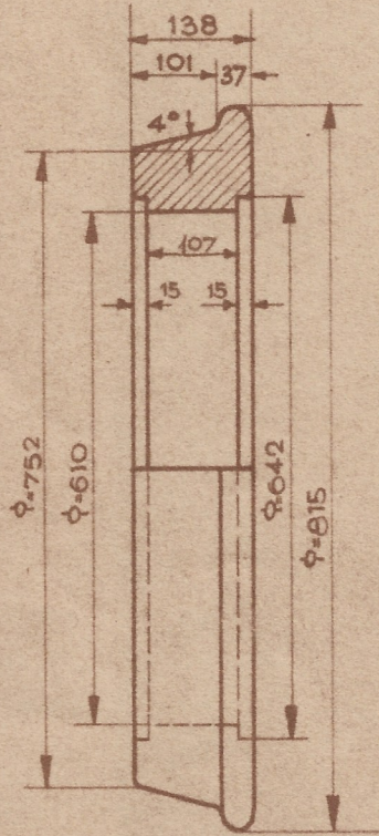
LOCALISAÇÃO DOS C.P. PARA ENSAIOS MECANICOS EM SECÇÃO TRANSVERSAL ESCALA 1:5
