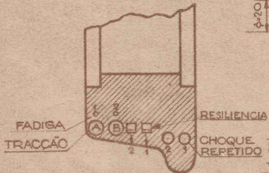
LOCALISAÇÃO DOS C.P. PARA ENSAIOS MECANICOS EM SECÇÃO TRANSVERSAL ESCALA 1:5
